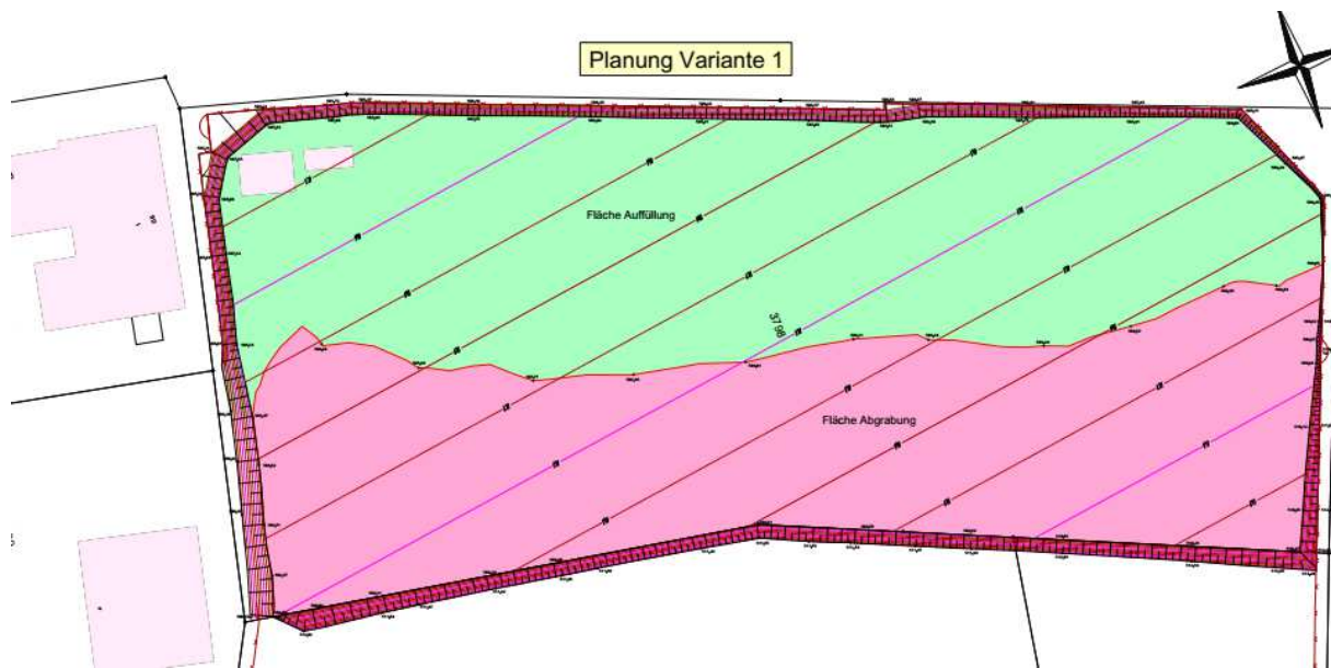
Abb. 14 Auszug der Planzeichnung zu geplanten Aufschüttungen und Abgrabungen – Ohne Maßstab
